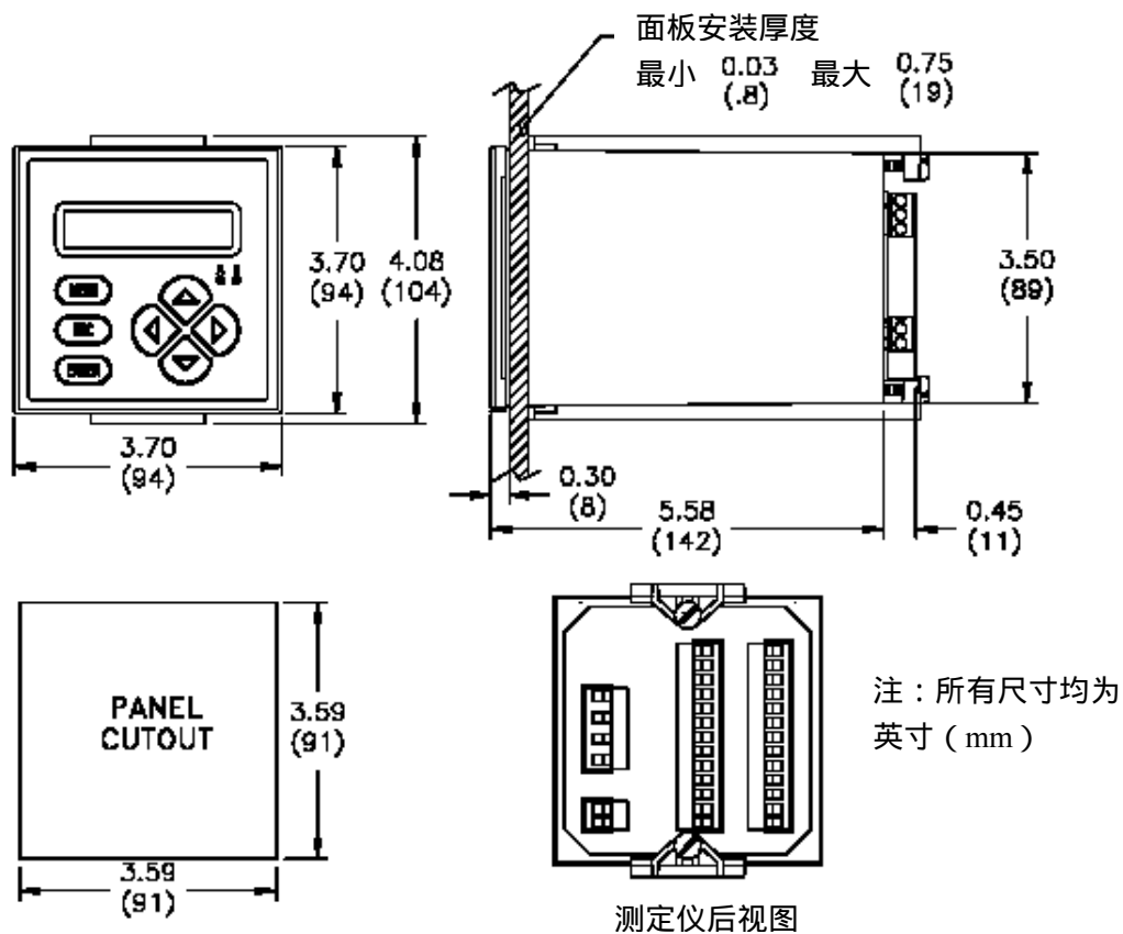
图 2-1 序列号中前缀为“A”的测定仪安装尺寸图
