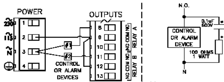
图 2-6 连接控制/报警装置到机电继电器(用于感应负载开关) * 推荐使用这些组件以得到最大的继电器寿命。为了得到最佳性能，这些组件应该尽可能安装最接近于负载的地方。
