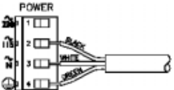
图 2-7 115V 单相电源的连接 (90~130 VAC)
