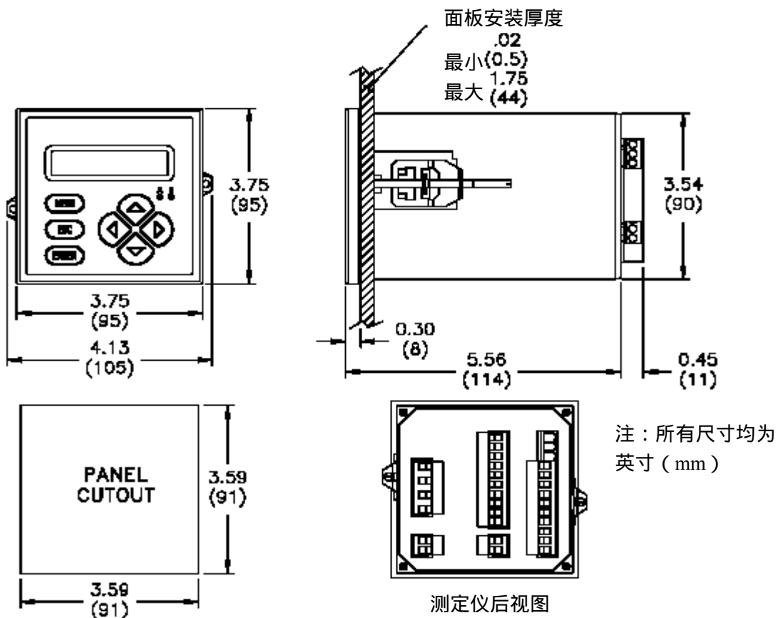
图 2-2 序列号中无前缀的测定仪安装尺寸图
