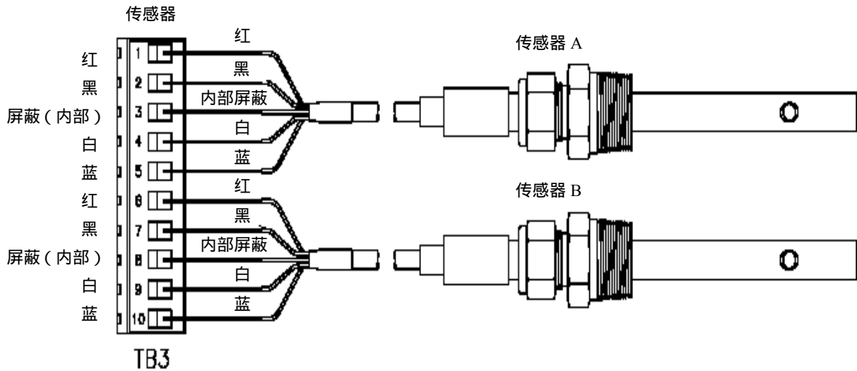
图 2-5 连接 GLI 性能改进型接触电导传感器
