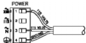
图 2-9 230V 分相电源的连接 (190~260 VAC)
