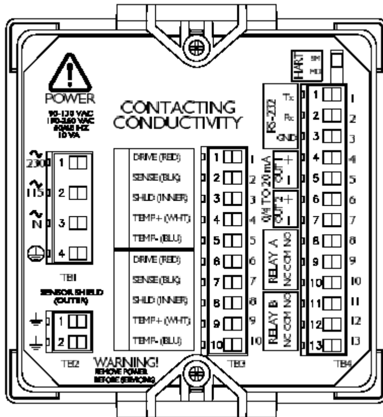
图 2-3 序列号中带“A”前缀的测定仪的接线图（HART 开关仅当选择了 HART 选项时有效）
